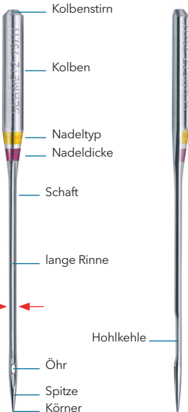
Vorderansicht
